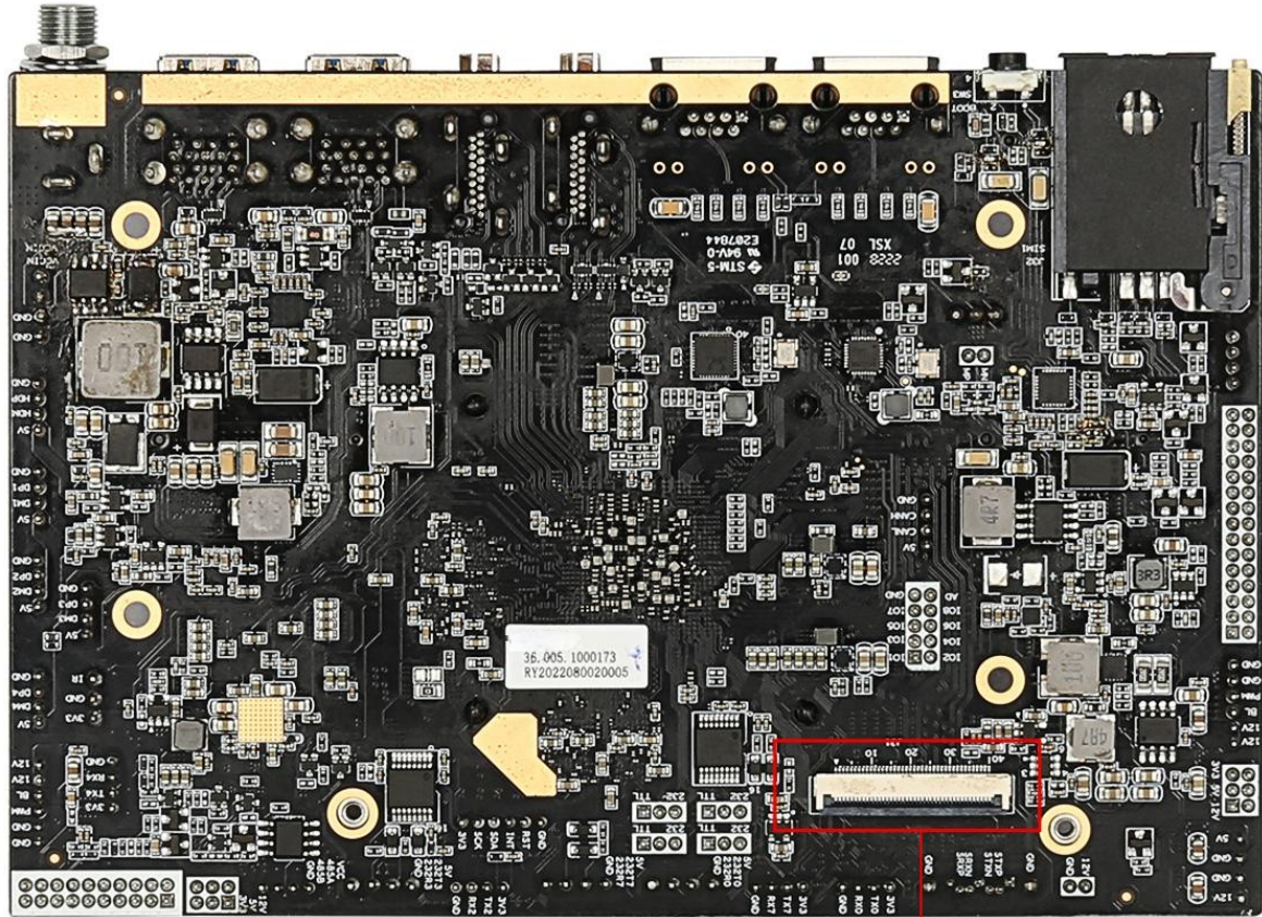
MIPI屏接口
