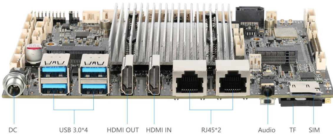
【Interface diagram】
